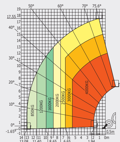
Погрузчик с выставленными стабилизаторами с вилами
